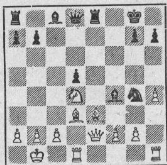
Stilling efter Hvids 18. Træk.
